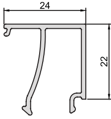
KOD-CODE CC-1240-13 TEORİK AĞIRLIK THEORETICAL WEIGHT 0,285 Kg/m
