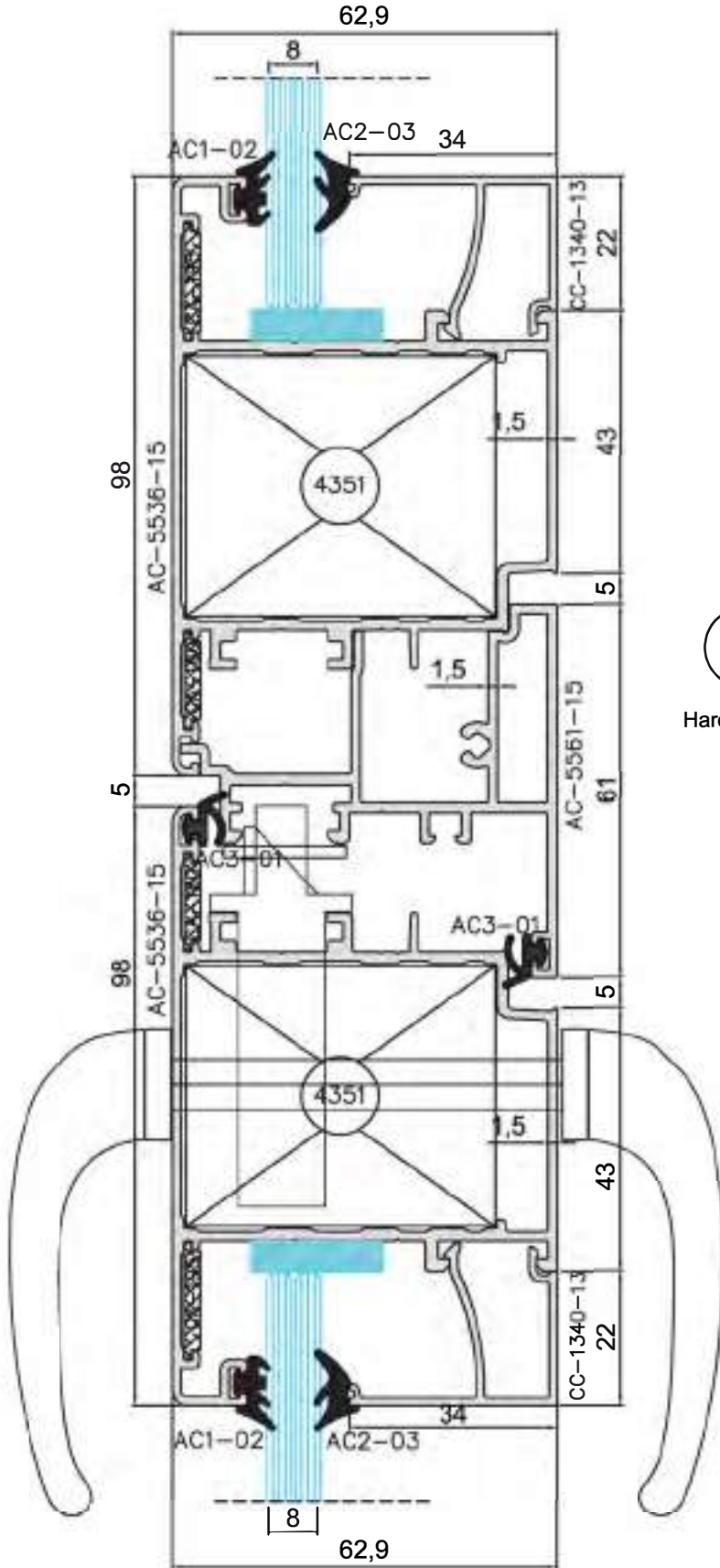
Dışa Açılım Çift Kanat Adaptörü
