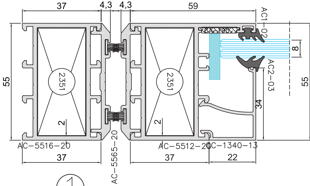
Dar Çarpma Kapı Kasa Detay
