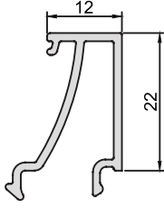
KOD-CODE CC-1120-13 TEORİK AĞIRLIK THEORETICAL WEIGHT 0,254 Kg/m
