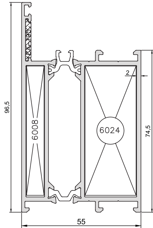
KOD-CODE AT-5514-20 TEORİK AĞIRLIK THEORETICAL WEIGHT 2,232 Kg/m
