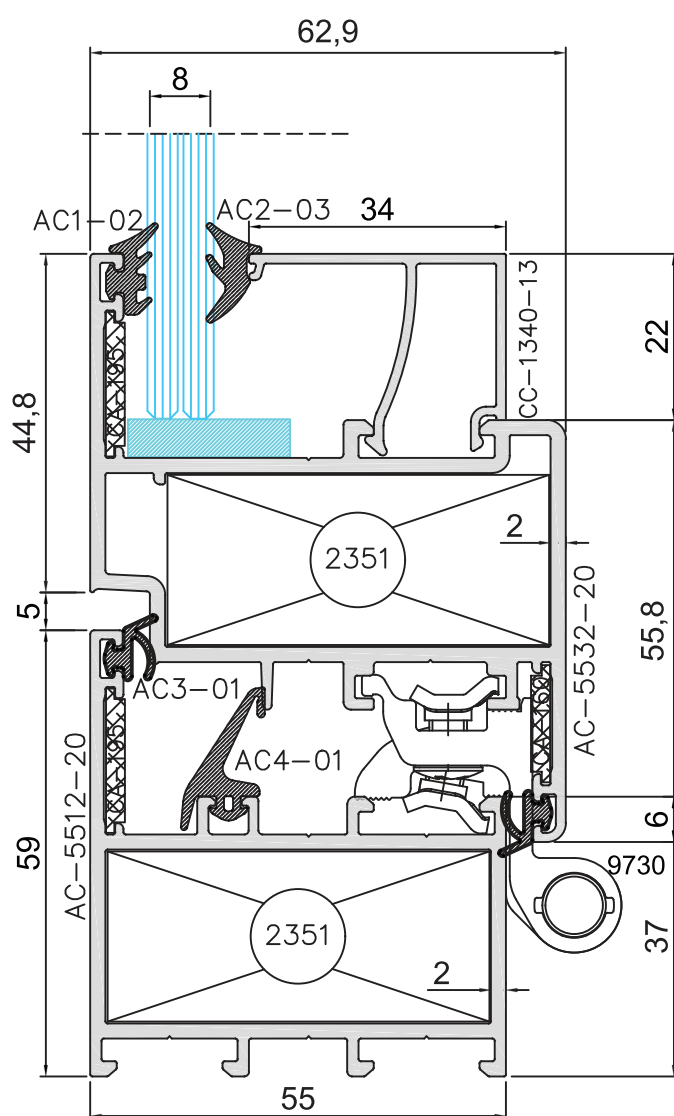
Menteşe Detay
