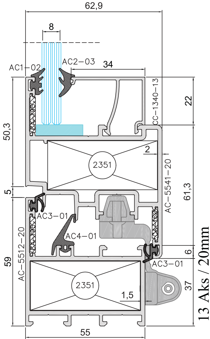
PVC 13Aks Menteşe Detay
