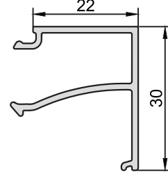
KOD-CODE CC-1300-13 TEORİK AĞIRLIK THEORETICAL WEIGHT 0,305 Kg/m
