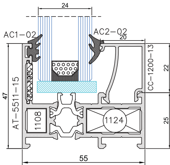
① Düz Kasa Detay
