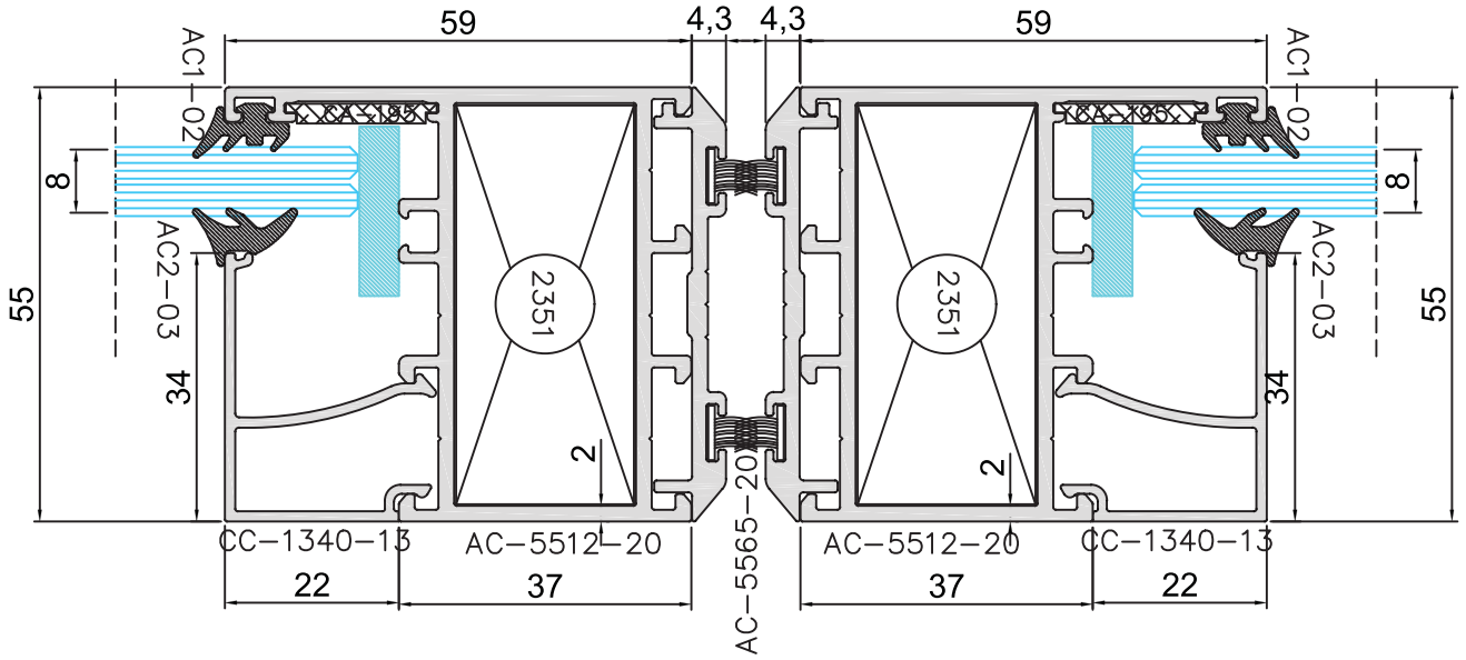
Dar Çarpma Kapı Kasa Detay
