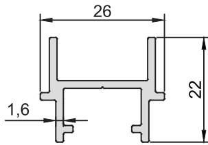
KOD-CODE ASL-6036-16 TEORİK AĞIRLIK THEORETICAL WEIGHT 0,324 Kg/m
