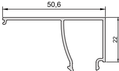
KOD-CODE CC-1400-13 TEORİK AĞIRLIK THEORETICAL WEIGHT 0,341 Kg/m
