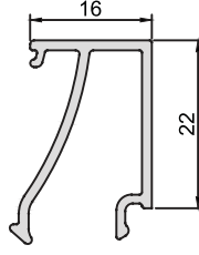
KOD-CODE CC-1160-13 TEORİK AĞIRLIK THEORETICAL WEIGHT 0,260 Kg/m
