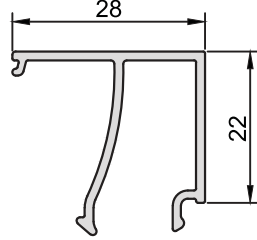
KOD-CODE CC-1280-13 TEORİK AĞIRLIK THEORETICAL WEIGHT 0,300 Kg/m
