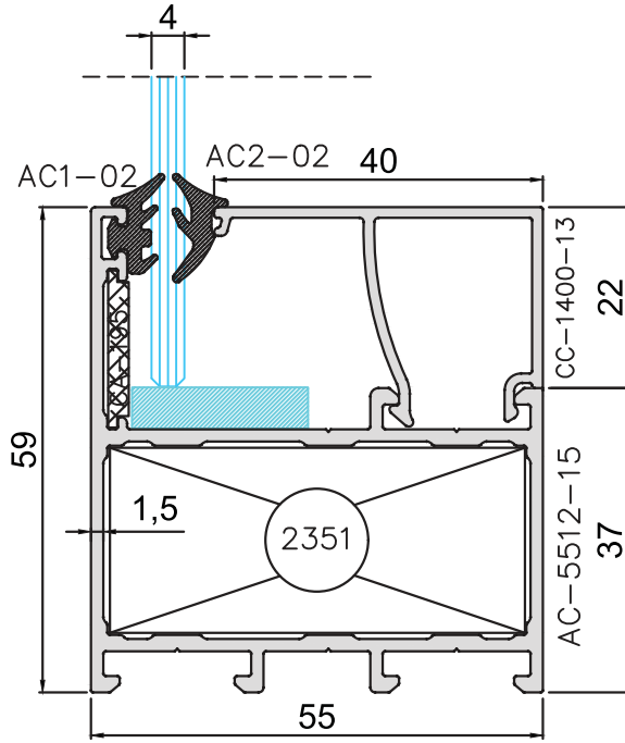
1 Düz Kasa Detay
