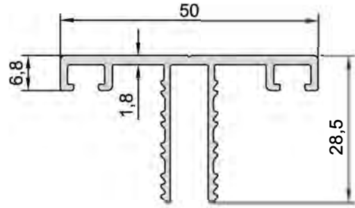
KOD-CODE 8509 TEORİK AĞIRLIK THEORETICAL WEIGHT 0,518 Kg/m
