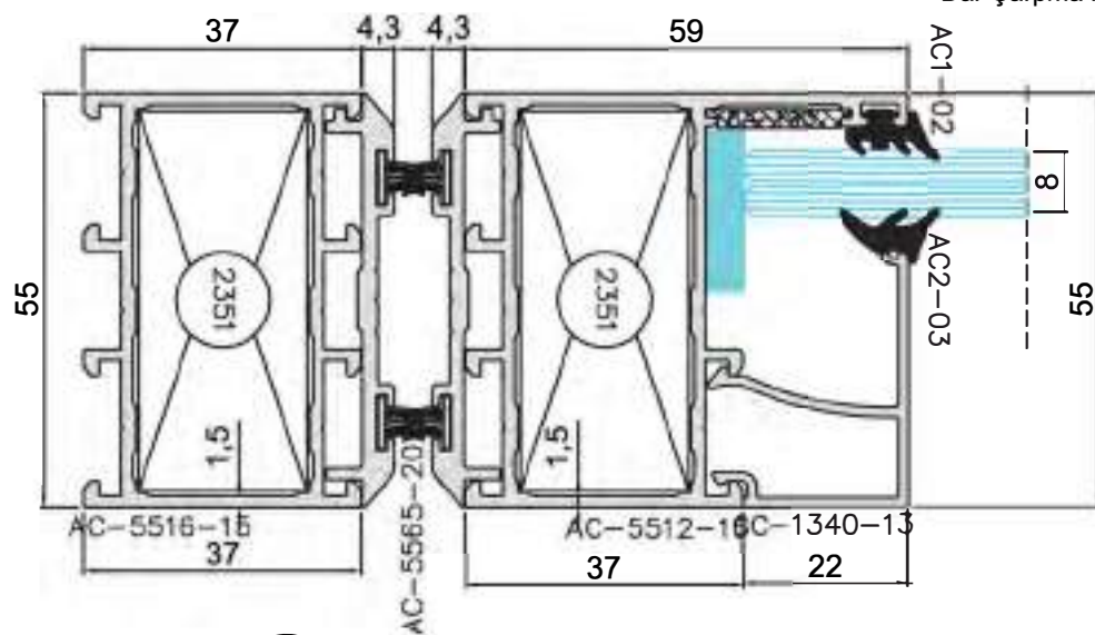
① Dar Çarpma Kapı Kasa Detay
