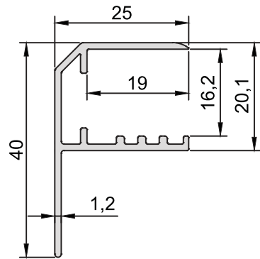
KOD-CODE 8508 TEORİK AĞIRLIK THEORETICAL WEIGHT 0,318 Kg/m
