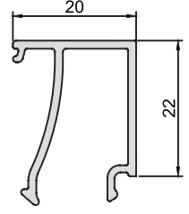
KOD-CODE CC-1200-13 TEORİK AĞIRLIK THEORETICAL WEIGHT 0,270 Kg/m
