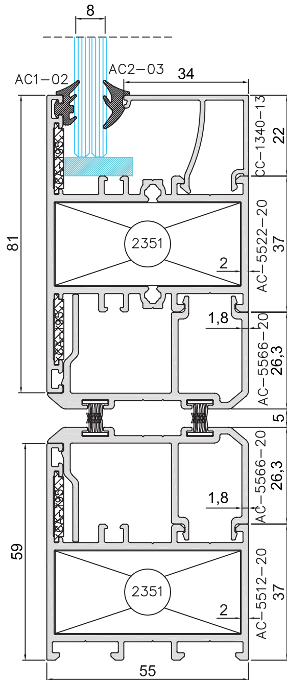
Geniş Çarpma Kapı Kasa Detay
