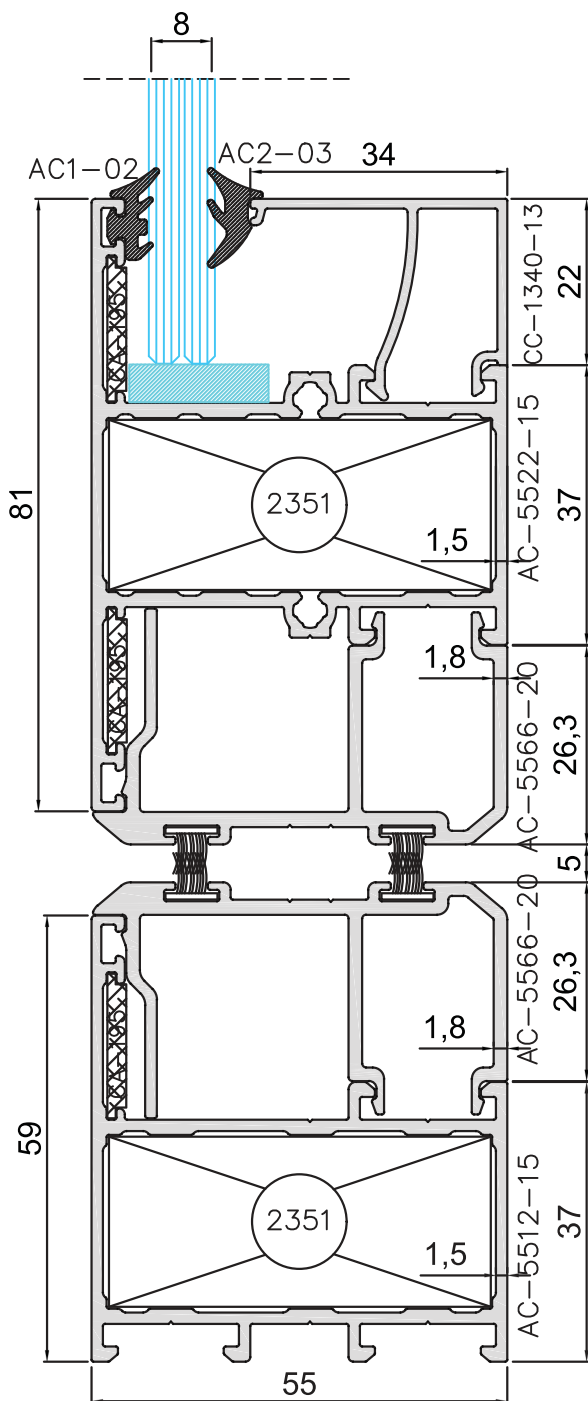
Geniş Çarpma Kapı Kasa Detay
