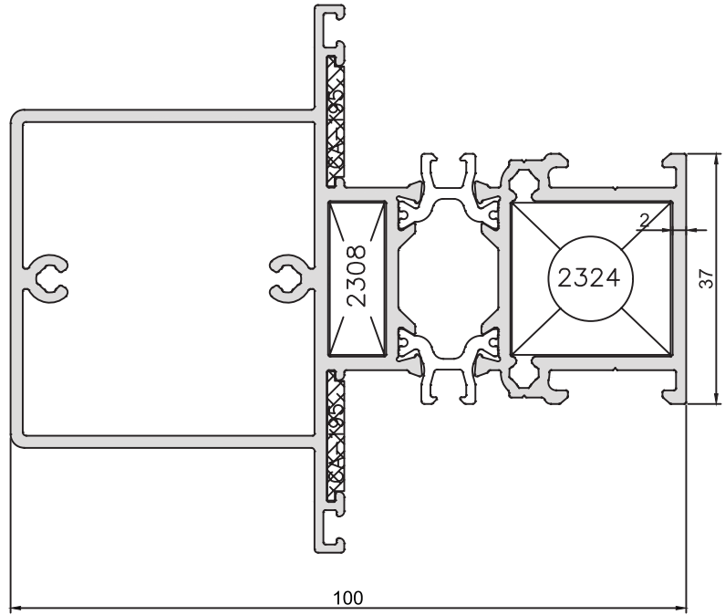
KOD-CODE AT-5526-20 TEORİK AĞIRLIK THEORETICAL WEIGHT 2,429 Kg/m
