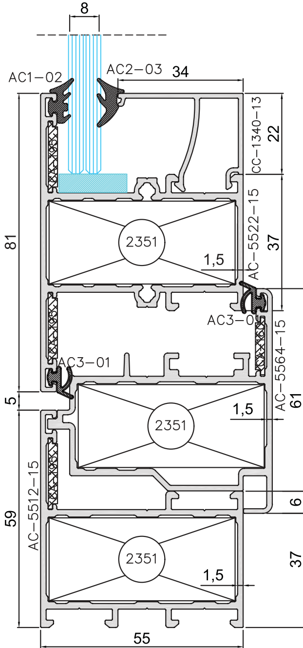
Pivot Menteşe Detay
