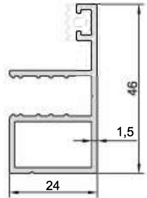
KOD-CODE 8511 TEORİK AĞIRLIK THEORETICAL WEIGHT 0,559 Kg/m
