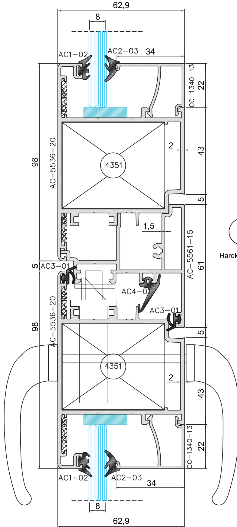
Dışa Açılım Çift Kanat Adaptörü
