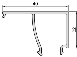
KOD-CODE CC-1400-13 TEORİK AĞIRLIK THEORETICAL WEIGHT 0,341 Kg/m
