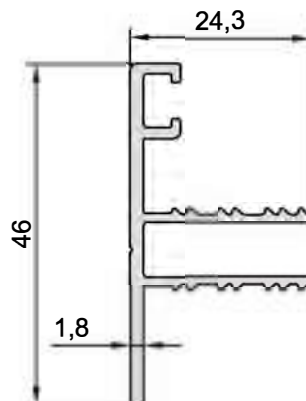
KOD-CODE 8510 TEORİK AĞIRLIK THEORETICAL WEIGHT 0,422 Kg/m
