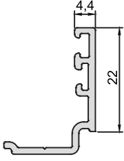
KOD-CODE CC-1044-13 TEORİK AĞIRLIK THEORETICAL WEIGHT 0,212 Kg/m
