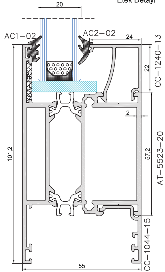
Etek Detayı
