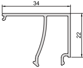
KOD-CODE CC-1340-13 TEORİK AĞIRLIK THEORETICAL WEIGHT 0,320 Kg/m
