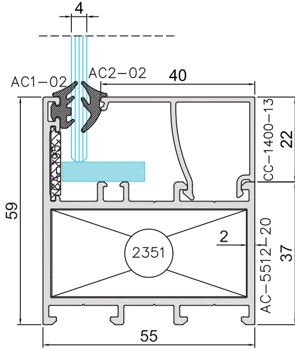
Düz Kasa Detay
