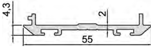
KOD-CODE AC-5565-20 TEORİK AĞIRLIK THEORETICAL WEIGHT 0,427Kg/m
