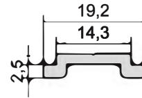
KOD-CODE 765 TEORİK AĞIRLIK THEORETICAL WEIGHT 0,138Kg/m
