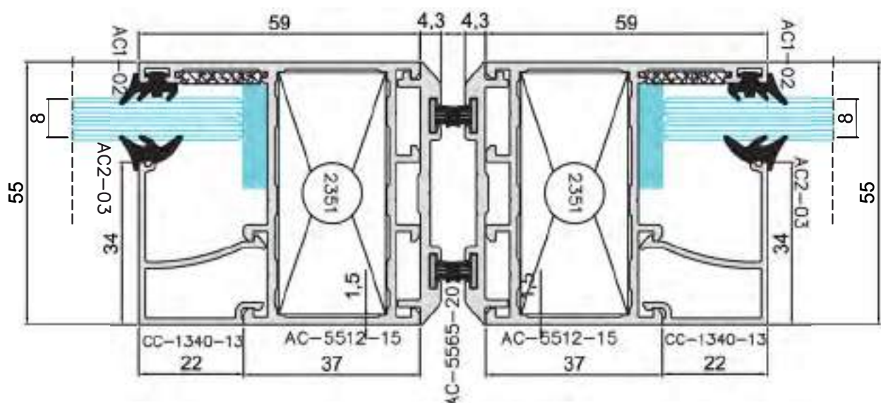
2 Dar Çarpma Kapı Kilit Detay
