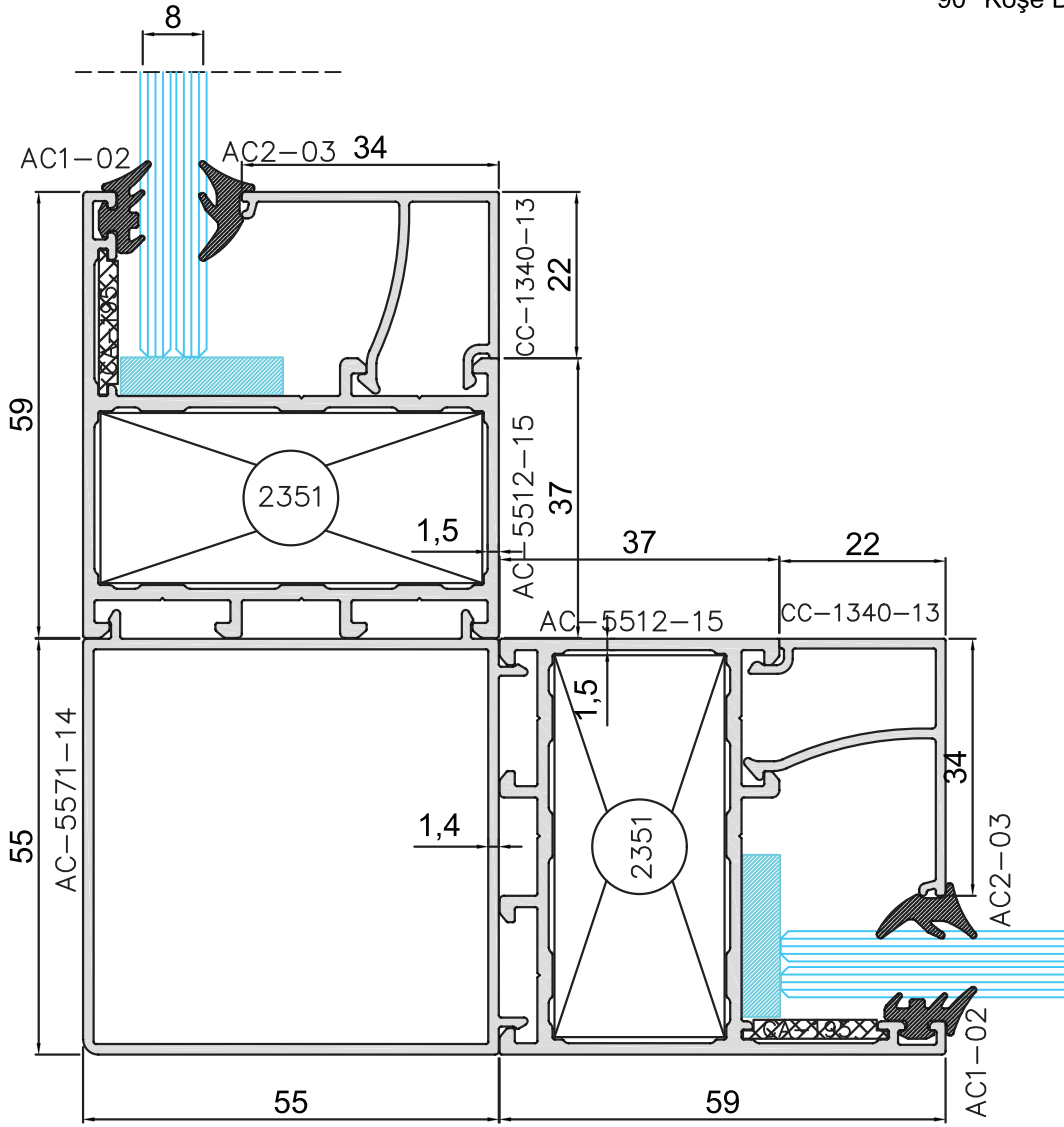
90° Köşe Dönüş
