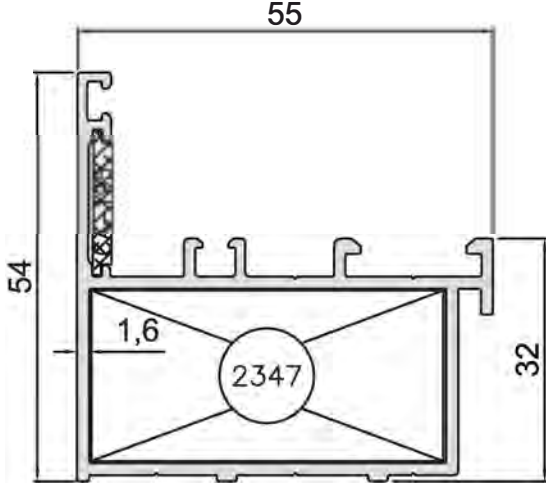
KOD-CODE AC-5563-16 TEORİK AĞIRLIK THEORETICAL WEIGHT 0,930Kg/m
