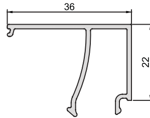
KOD-CODE CC-1360-13 TEORİK AĞIRLIK THEORETICAL WEIGHT 0,327 Kg/m
