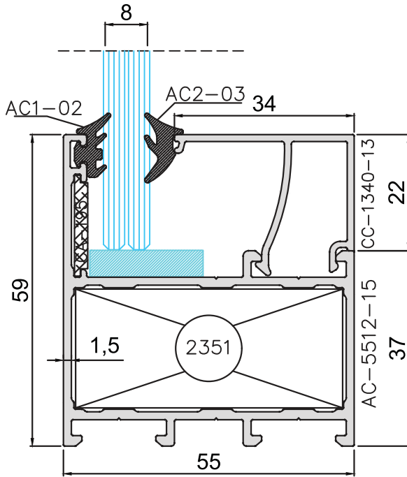
1 Düz Kasa Detay
