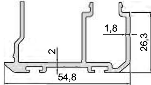
KOD-CODE AC-5566-20 TEORİK AĞIRLIK THEORETICAL WEIGHT 0,761Kg/m
