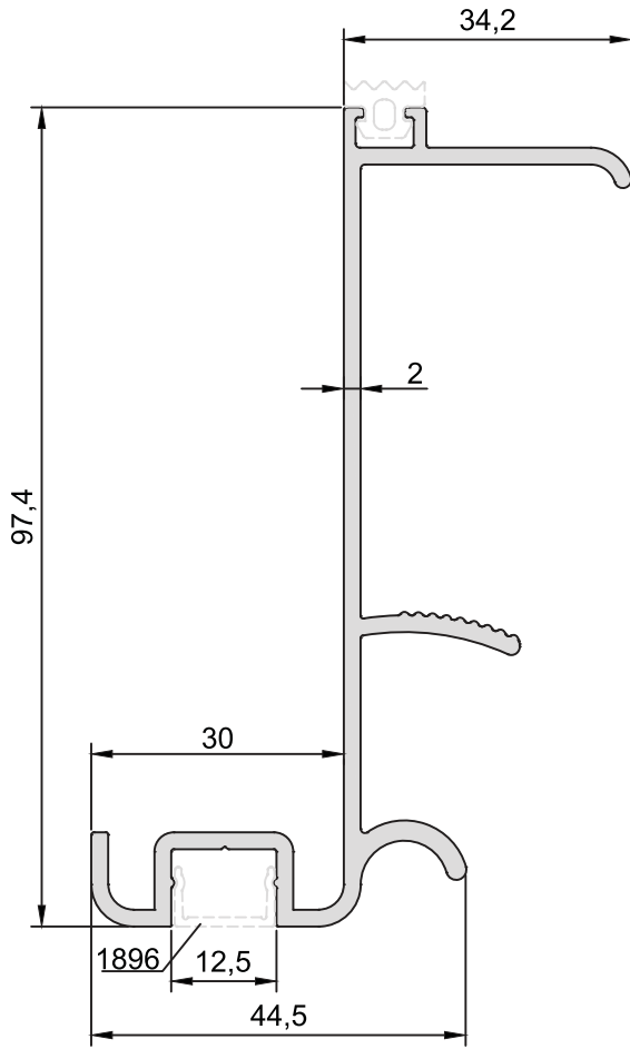
KOD-CODE 8505 TEORİK AĞIRLIK THEORETICAL WEIGHT 1,236 Kg/m
